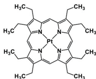
PtOEP
