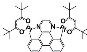
(dbx)((dpm)Pt) 2
