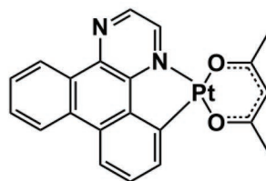
(dbx)Pt(acac)
